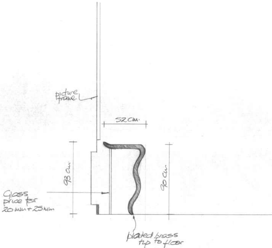
SIDE ELEVATION - TERRAZZO TABLE
